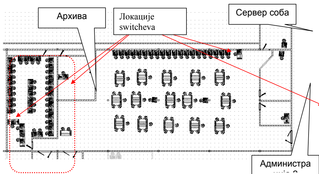
Слика број 14. – Тлоцрт просторија у ГЦБ
